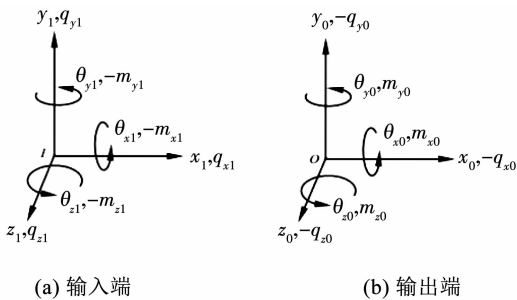
图 3 坐标系及符号约定
