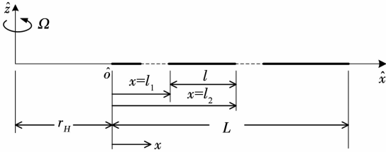
图4 旋转梁挥舞方向振动的符号约定和坐标系
