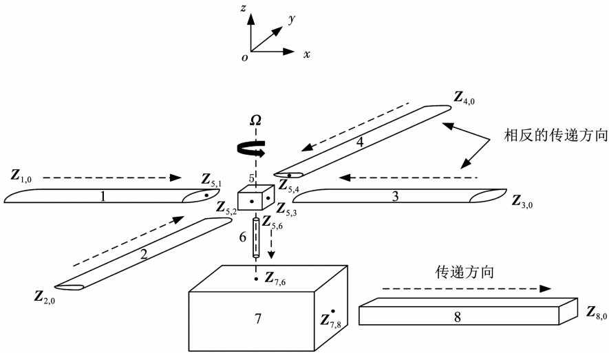
图 2 直升机拓扑模型 Fig. 2 Helicopter topology model
